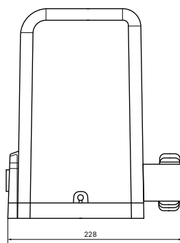
Розміри NAVI 1000/1500
