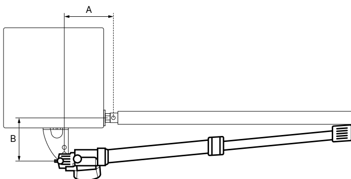
Монтажні розміри SW 4000 / SW 6000
