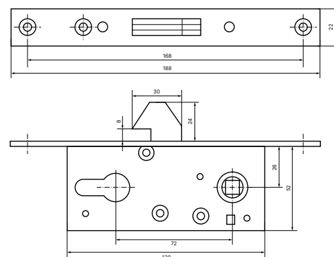
Креслення К-60
