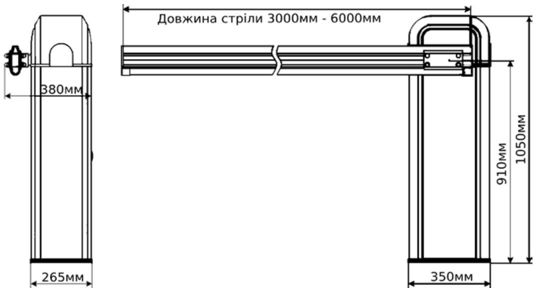
Розміри шлагбауму 306 DC
