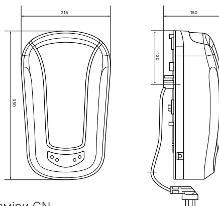
Розміри GN
