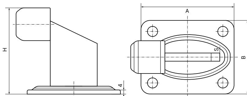
Розміри MX04A / MX04B
