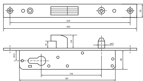
Креслення К-40
