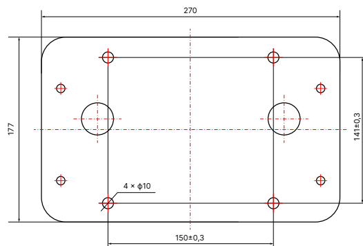
Монтажні розміри NAVI 1000/1500
