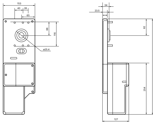
Розміри SFO
