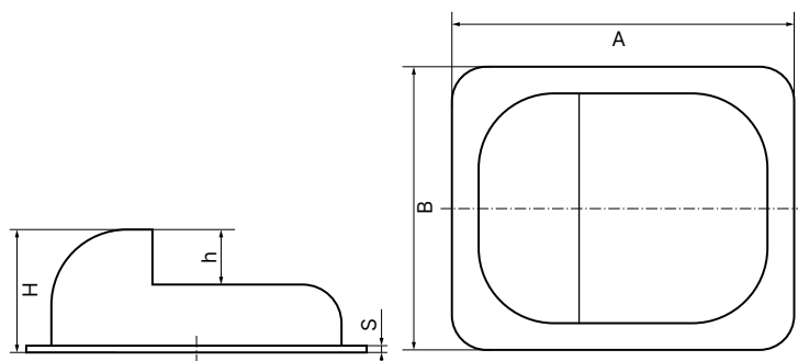
Розміри MX05A / MX05B
