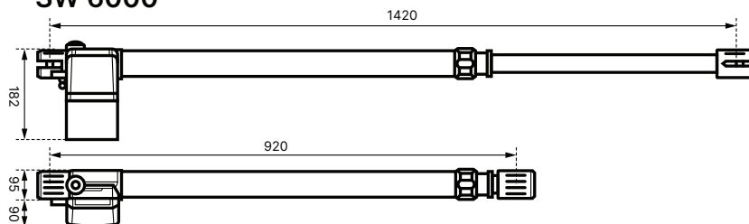
Розміри SW 4000 / SW 6000
