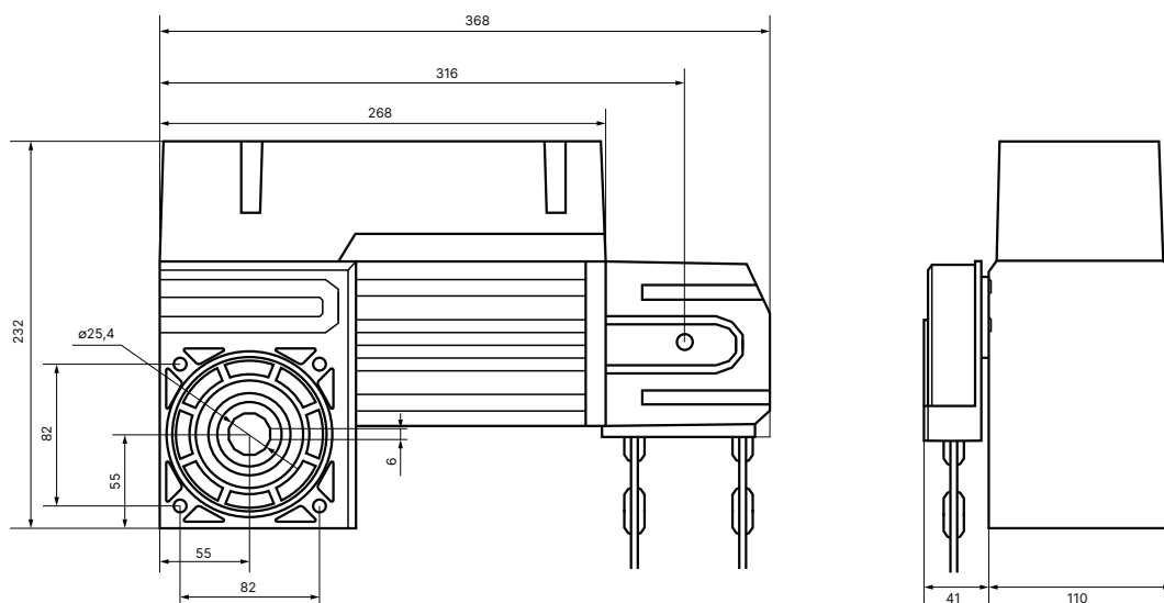
Розміри IND LCD
