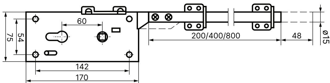
Креслення замку KS-5
