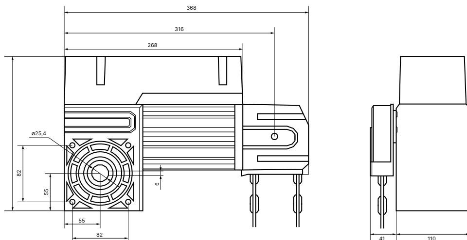
Розміри IND
