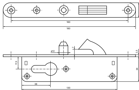
Креслення К-35
