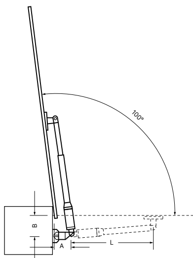
Монтажні розміри ANT SW
