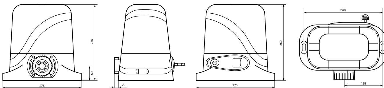
Розміри ANT
