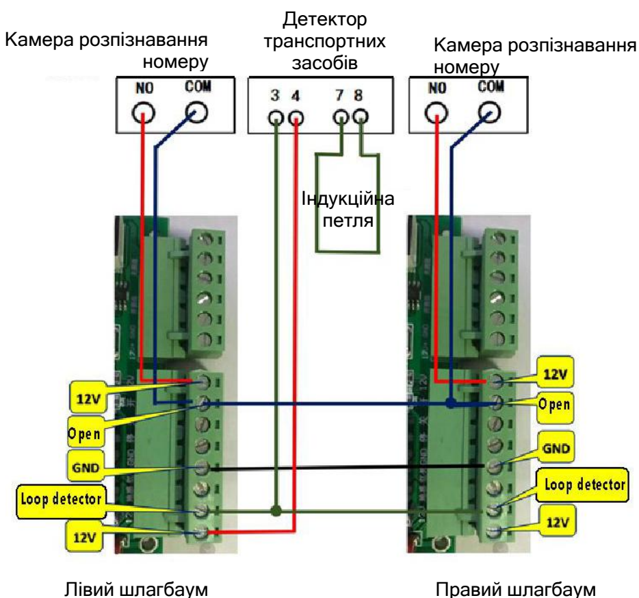
Схема підключення шлагбаумів
