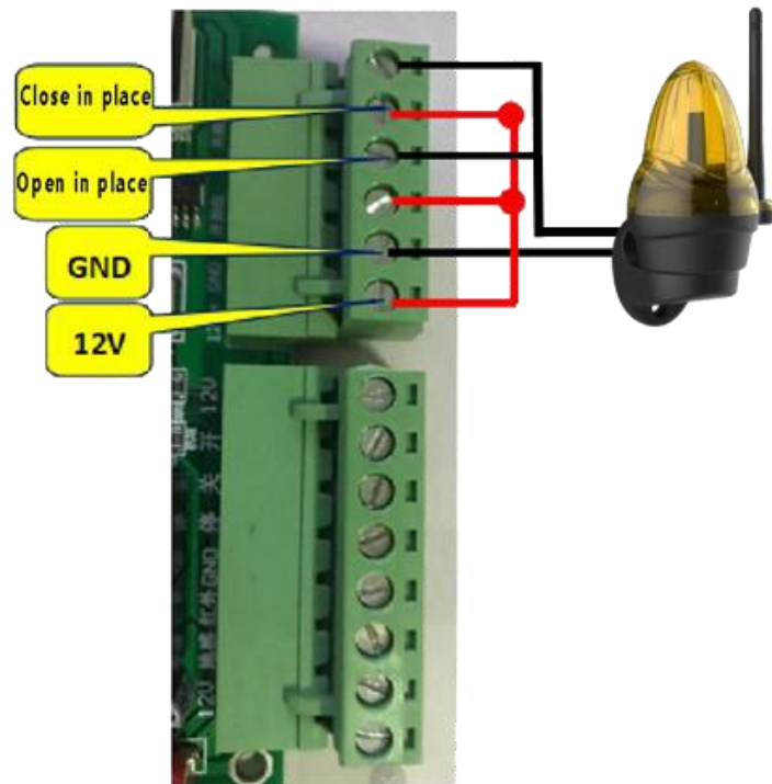
Схема підключення сигнальної лампи
